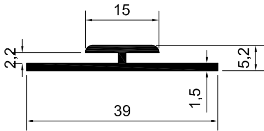
KOD-7006 TEORİK AĞIRLIK-0,225 KG/M
