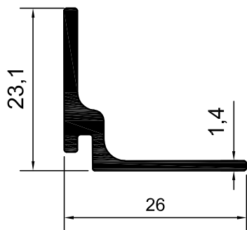
KOD-1117 TEORİK AĞIRLIK-0,247 KG/M
