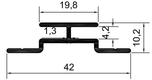
KOD-1028 TEORİK AĞIRLIK-0,252 KG/M
