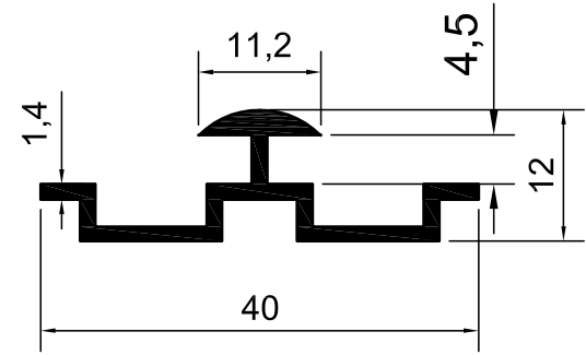
KOD-1420 TEORİK AĞIRLIK- 0,269 KG/M
