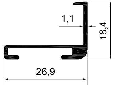
KOD-1112 TEORİK AĞIRLIK-0,187 KG/M
