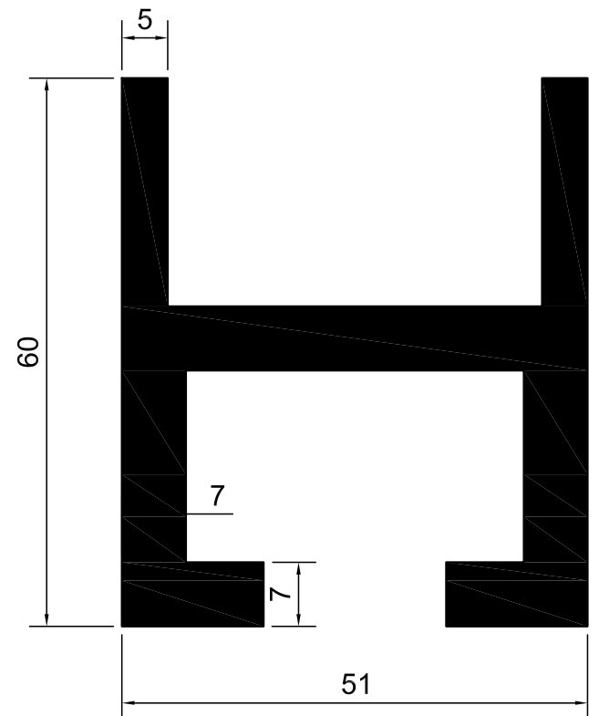
KOD-7067 TEORİK AĞIRLIK-3,029 KG/M
