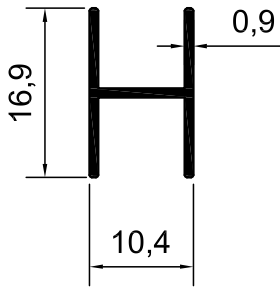
KOD-1412 TEORİK AĞIRLIK- 0,103 KG/M
