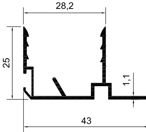
KOD-7021 TEORİK AĞIRLIK-0,328 KG/M
