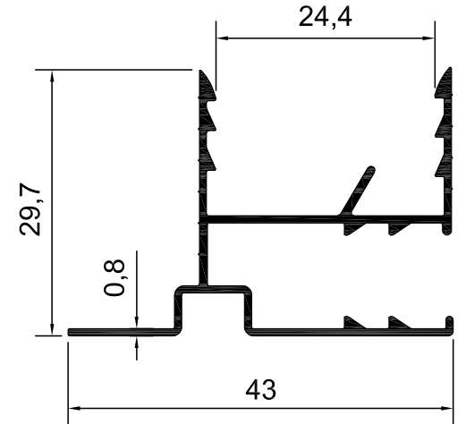
KOD-7022 TEORİK AĞIRLIK-0,312 KG/M
