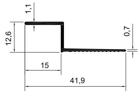
KOD-1119 TEORİK AĞIRLIK-0,139 KG/M
