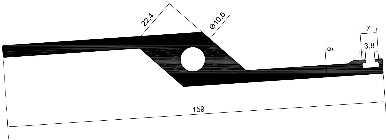
KOD-7064 TEORİK AĞIRLIK-3,164 KG/M
