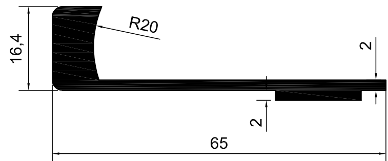
KOD-7066 TEORİK AĞIRLIK-0,764 KG/M
