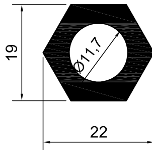
KOD-8507 TEORİK AĞIRLIK-0,558 KG/M
