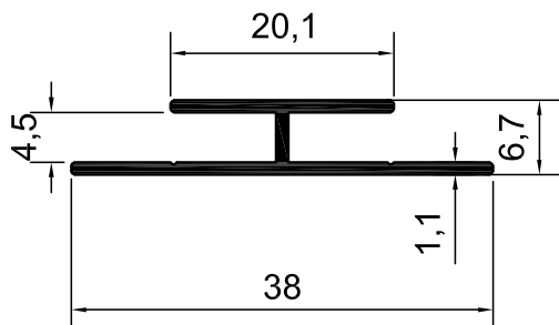
KOD-1410 TEORİK AĞIRLIK-0,185 KG/M
