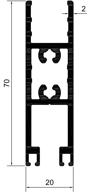
KOD-5400 TEORİK AĞIRLIK-1,233 KG/M
