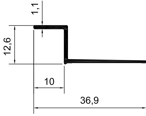
KOD-1120 TEORİK AĞIRLIK-0,125 KG/M
