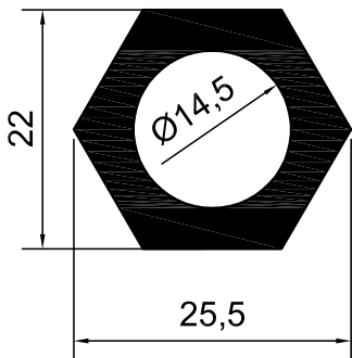
KOD-8506 TEORİK AĞIRLIK- 0,691 KG/M
