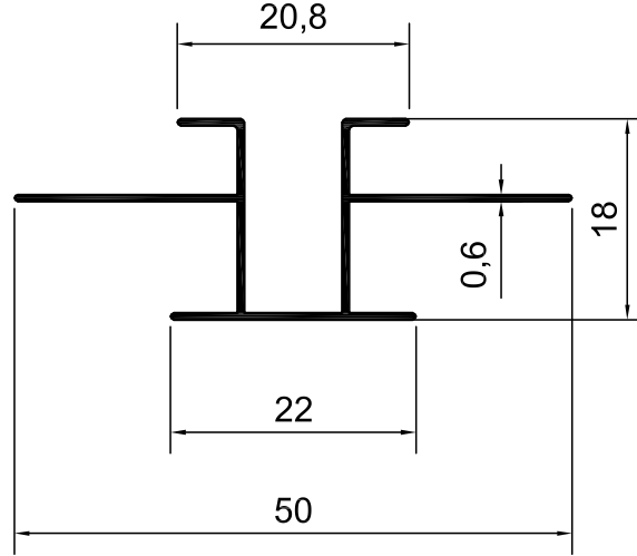
KOD-7039 TEORİK AĞIRLIK-0,176 KG/M
