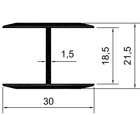
KOD-1416 TEORİK AĞIRLIK-0,294 KG/M
