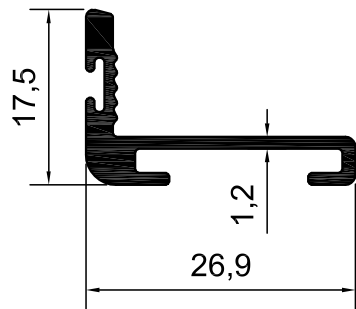
KOD-1111 TEORİK AĞIRLIK-0,239 KG/M
