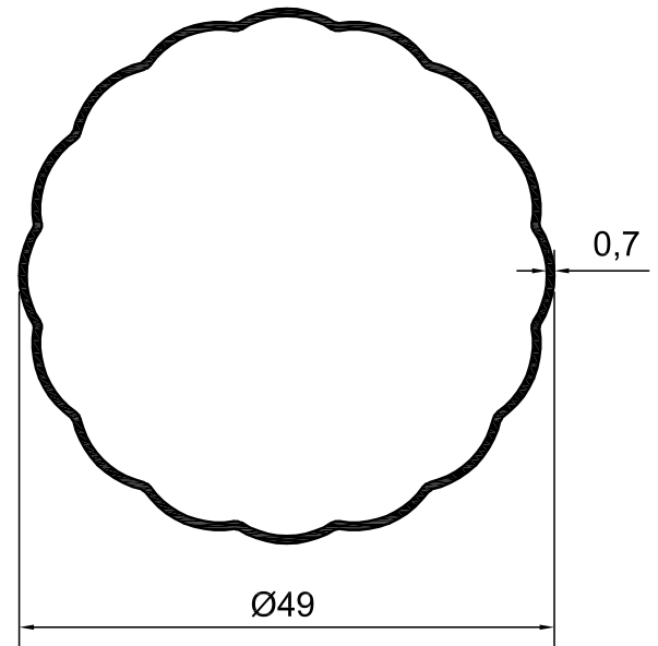
KOD-7041 TEORİK AĞIRLIK-0,290 KG/M
