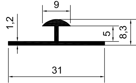
KOD-1419 TEORİK AĞIRLIK-0,153 KG/M
