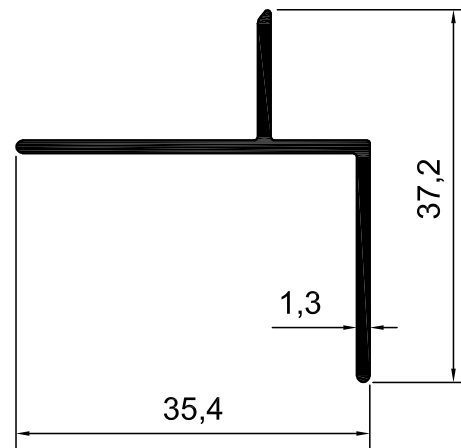
KOD-1118 TEORİK AĞIRLIK-0,249 KG/M
