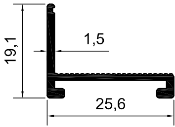
KOD-1300 TEORİK AĞIRLIK-0,197 KG/M
