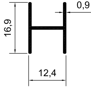
KOD-1413 TEORİK AĞIRLIK- 0,108 KG/M
