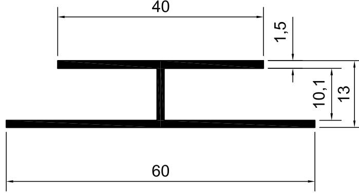
KOD-1417 TEORİK AĞIRLIK-0,428 KG/M
