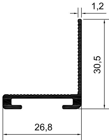
KOD-1113 TEORİK AĞIRLIK-0,236 KG/M
