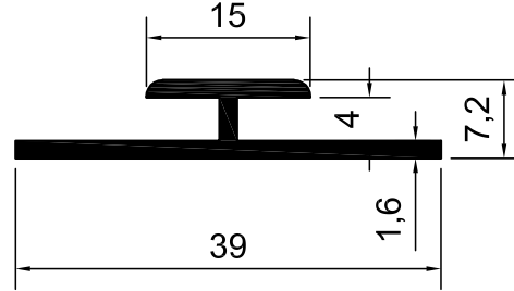
KOD-7007 TEORİK AĞIRLIK-0,248 KG/M
