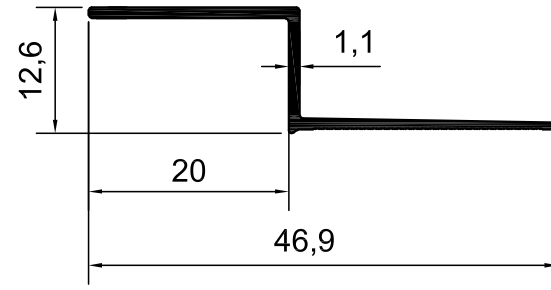
KOD-1121 TEORİK AĞIRLIK-0,138 KG/M
