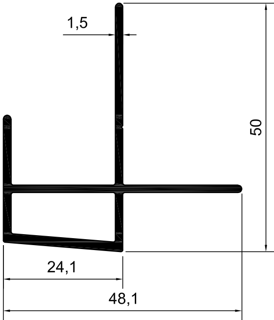
KOD-7040 TEORİK AĞIRLIK-0,598 KG/M
