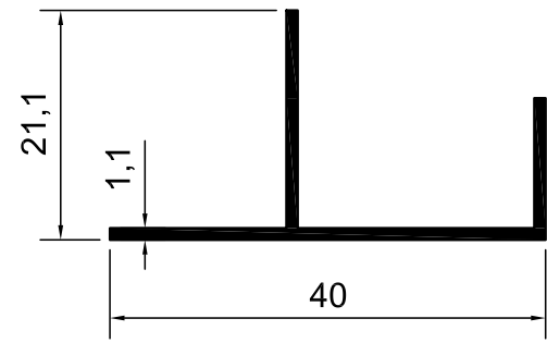
KOD-1124 TEORİK AĞIRLIK-0,210 KG/M
