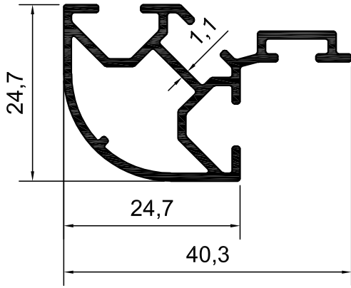
KOD-14644 TEORİK AĞIRLIK-1,000 KG/M
