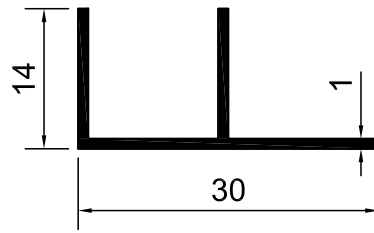
KOD-1123 TEORİK AĞIRLIK-0,152 KG/M
